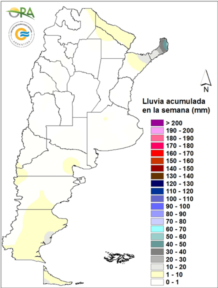
Precipitaciones acumuladas en la semana del 03/07/2024 al 09/07/2024
